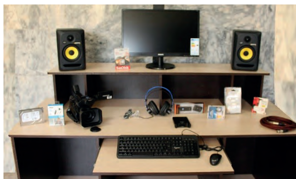
Таҷҳизот барои мини-студия Оборудование для мини-студии
